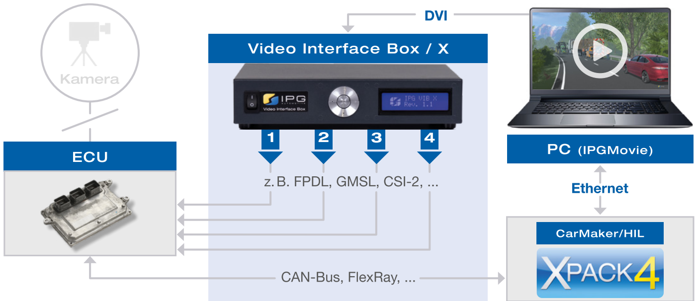
Schematische Darstellung des HIL-Aufbaus mit Video Interface Box / Video Interface Box X
